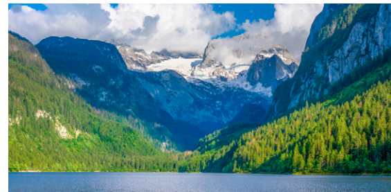
Die LINZ AG nutzt den Weltwassertag, um über den Schutz der wertvollen Ressource zu informieren. Im Bild: der Dachstein, dessen Gletscher immer mehr schwindet.
